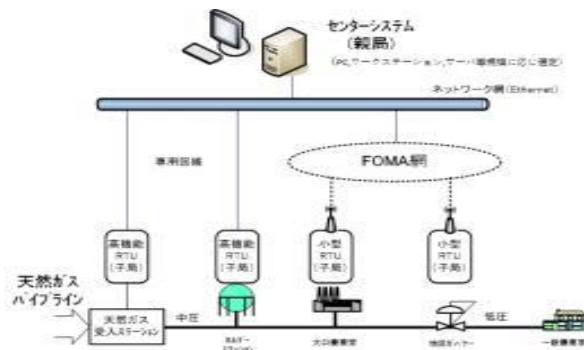
図1 都市ガス防災・供給監視システム構成イメージ
